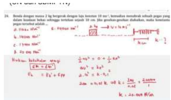
Gambar 1. Hasil analisis jawaban konsep usaha dan energi
